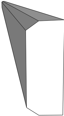
A4 (2x) 18x62x1831mm
